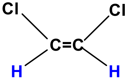
cis -1,2-dikloreten
