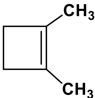
1,2-dimetil-1-siklobüten
