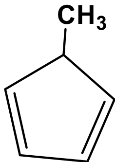
5-metil-1,3-siklopentadien
