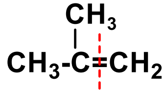
2-metilpropen
