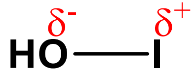
hipoiyodöz asit
