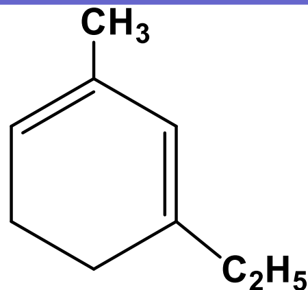
1-etil-3-metil-1,3-sikloheksadien
