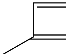
2-metil-1,3-bütadien
